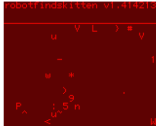
Figure 10.15.: Robotfindskitten
