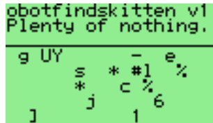
Figure 11.14.: Robotfindskitten
