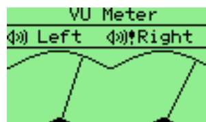
Figure 11.37.: VU-Meter
