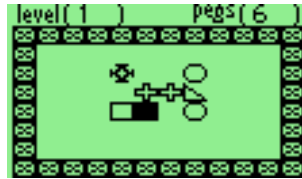
Figure 10.10: pegbox
