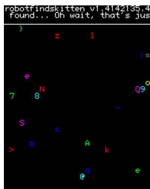
Figure 12.19.: Robotfindskitten
