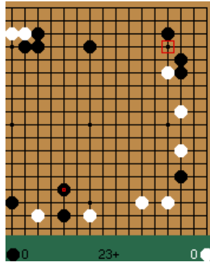
Figure 12.10.: Goban
