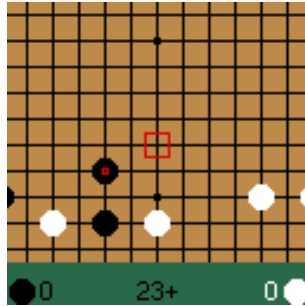
Figure 12.10.: Goban
