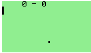
Figure 10.10.: Pong
