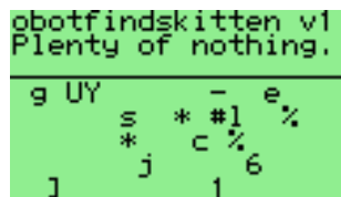
Figure 9.11.: Robotfindskitten
